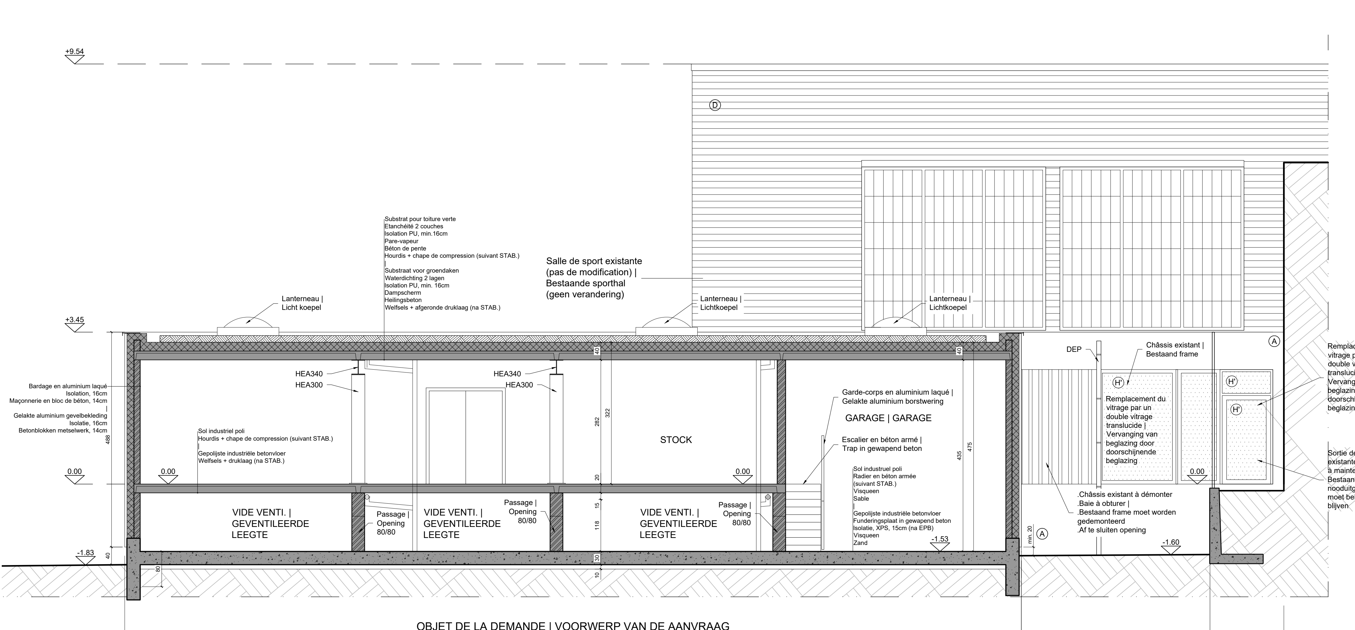
3.02 COUPE | DOORSNEDE - CC échelle / schaal : 1/50
