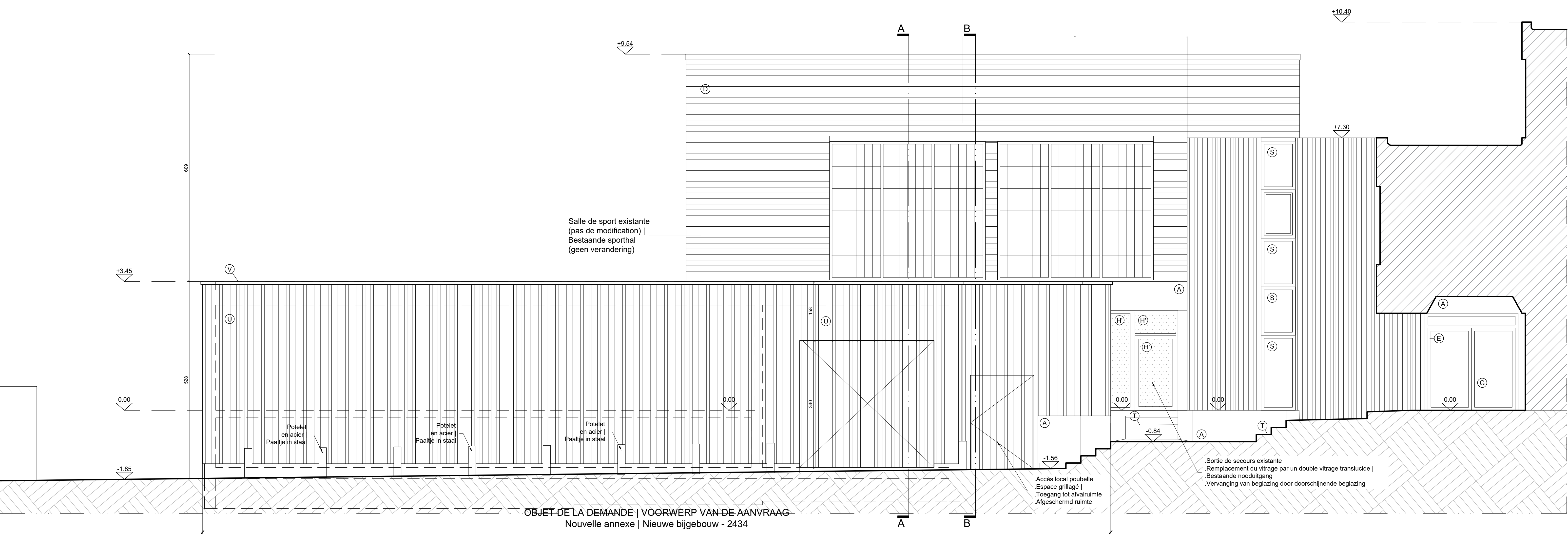
3.01 ELEVATION NORD | NOORDGEVEL échelle / schaal : 1/50
