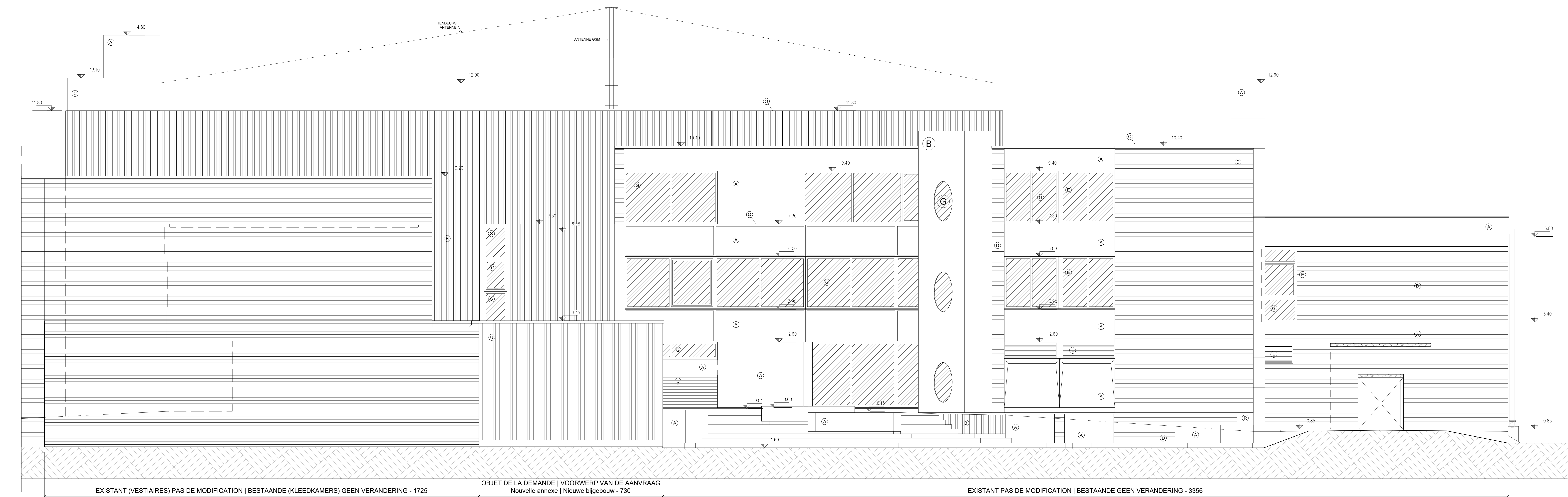
3.03 ELEVATION EST | OOSTGEVEL échelle / schaal : 1/50
