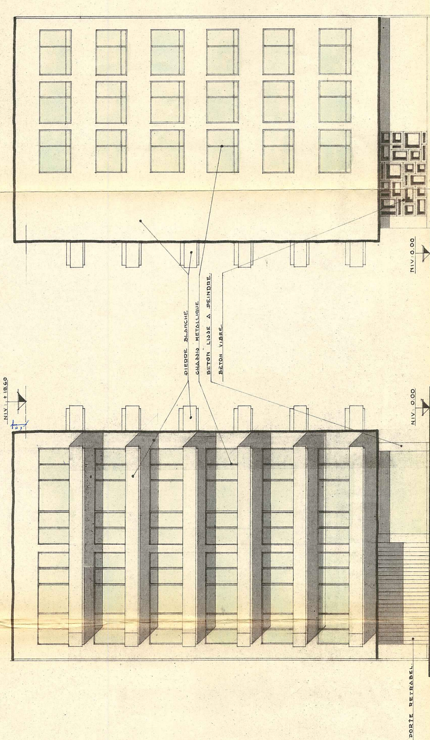
FACADE NORD - OUEST.
